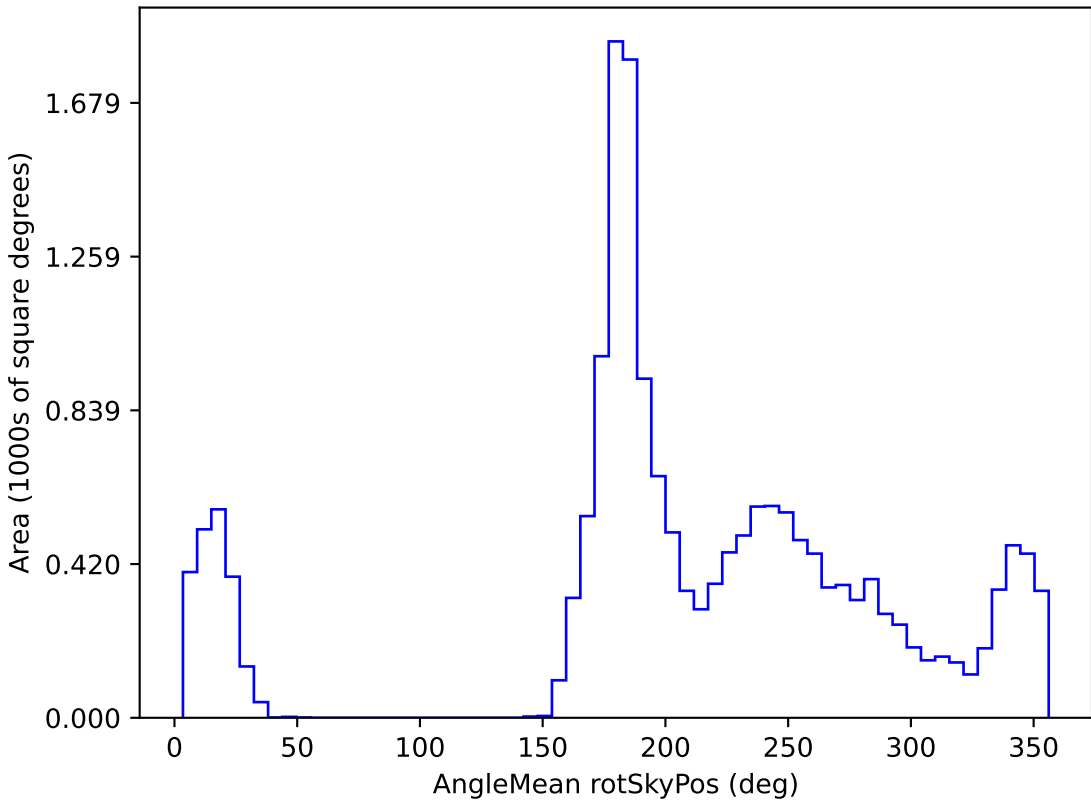
weather_cloudso4v3.4_10yrs WFD z band: AngleMean rotSkyPos
