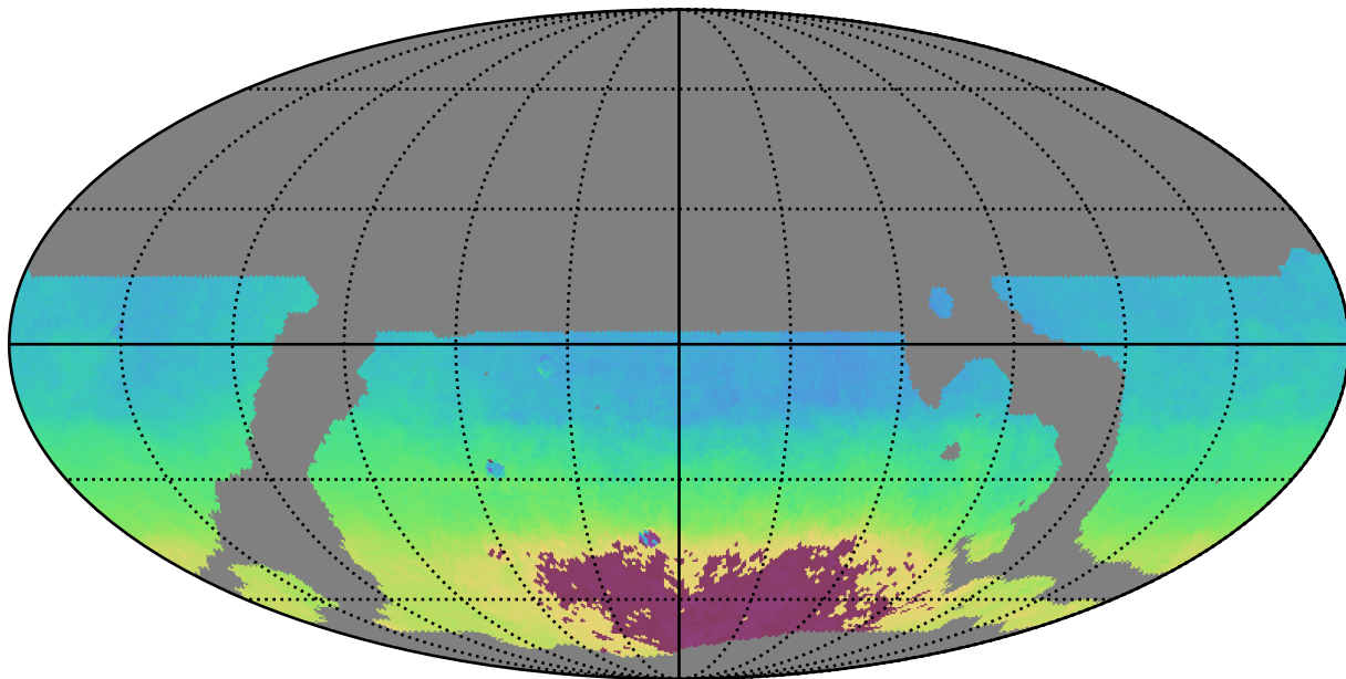
weather_cloudso4v3.4_10yrs WFD y band: AngleMean rotSkyPos
