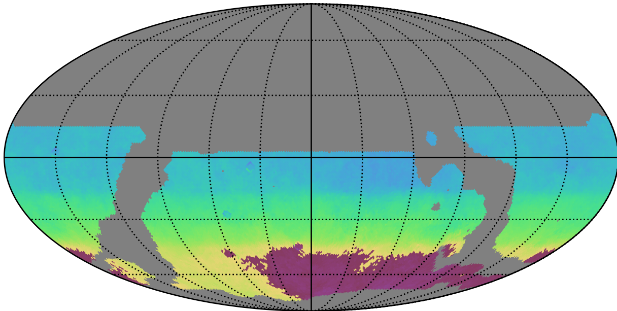
weather_cloudso4v3.4_10yrs WFD i band: AngleMean rotSkyPos
