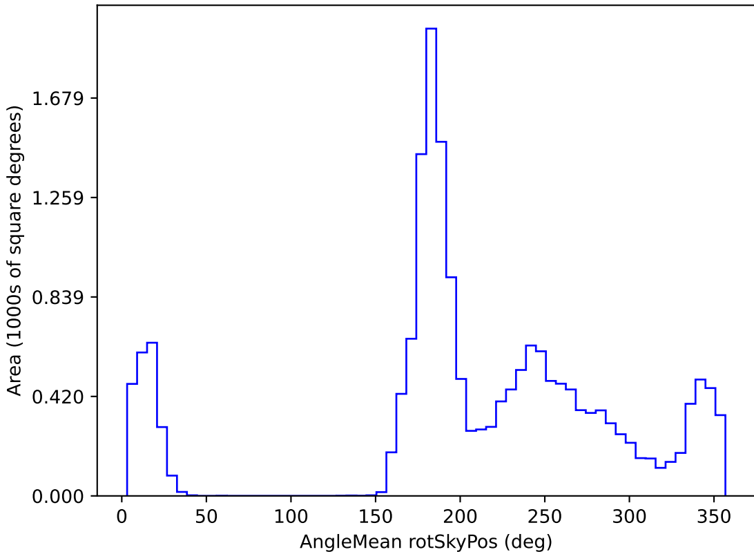
weather_cloudso4v3.4_10yrs WFD i band: AngleMean rotSkyPos
