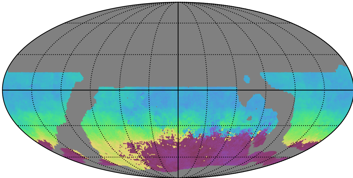
weather_cloudso4v3.4_10yrs WFD g band: AngleMean rotSkyPos
