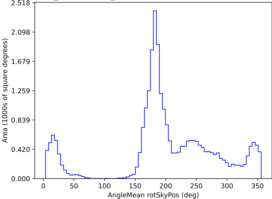
weather_cloudso4v3.4_10yrs All sky z band: AngleMean rotSkyPos
