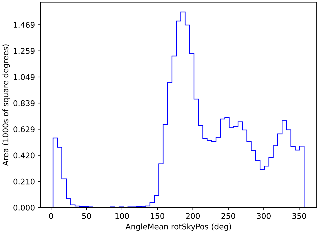
weather_cloudso4v3.4_10yrs All sky y band: AngleMean rotSkyPos
