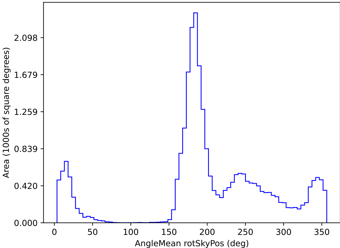
weather_cloudso4v3.4_10yrs All sky i band: AngleMean rotSkyPos
