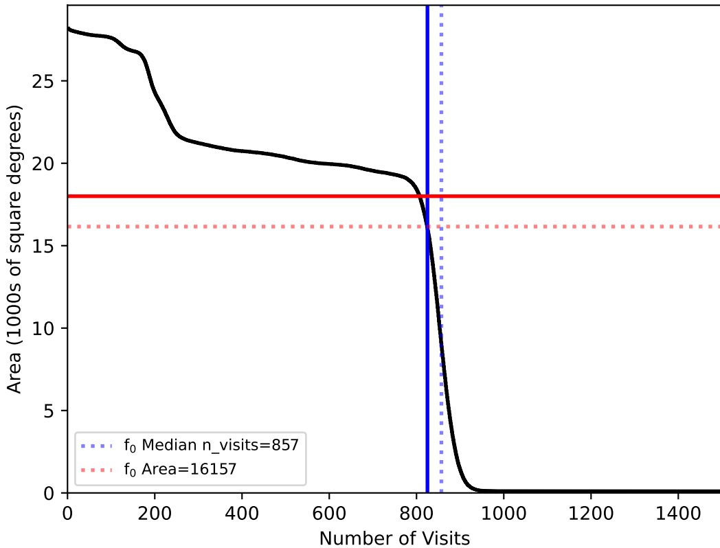
weather_cloudso4v3.4_10yrs : f0
