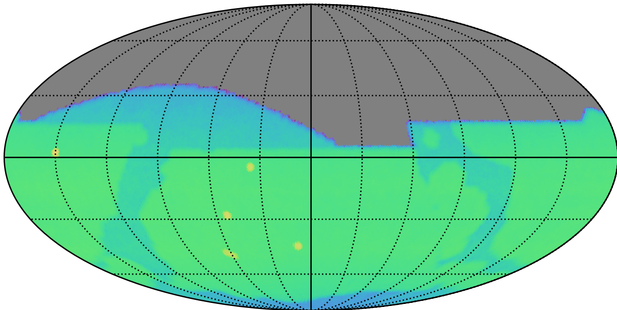
weather_cloudso4v3.4_10yrs i: CoaddM5
