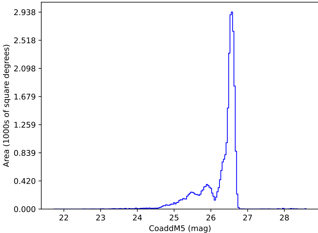
weather_cloudso4v3.4_10yrs i: CoaddM5
