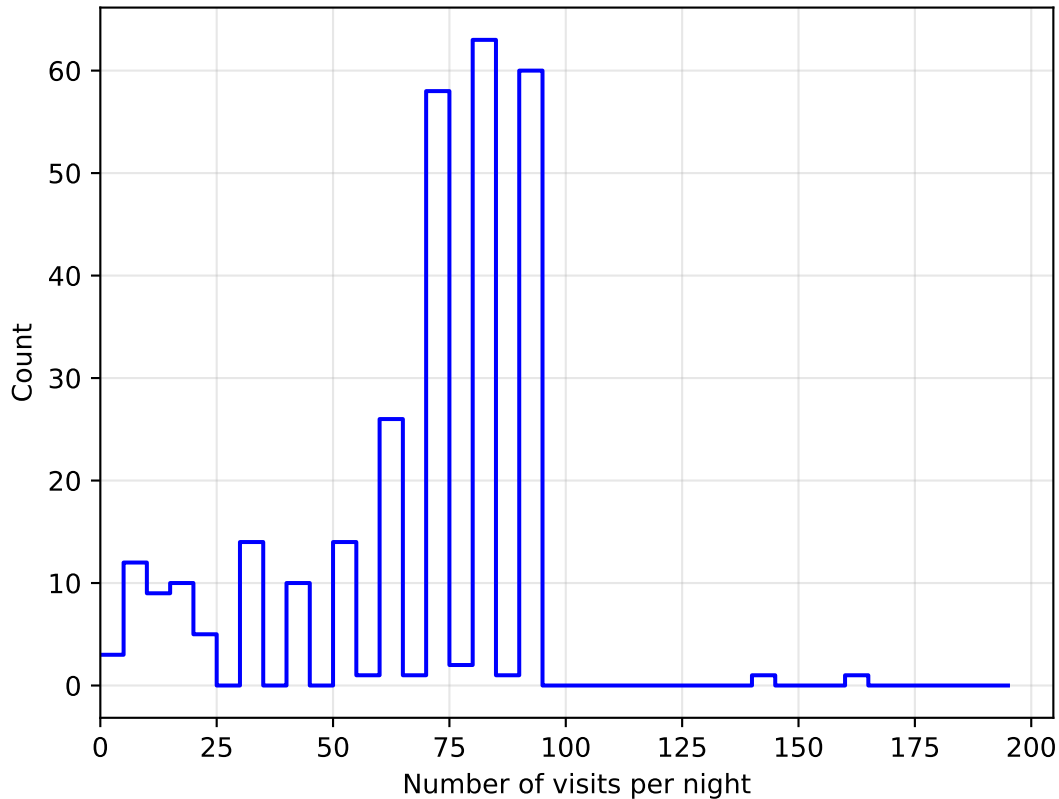
weather_cloudso4v3.4_10yrs all bands: DD:ELAISS1 NVisitsPerNight
