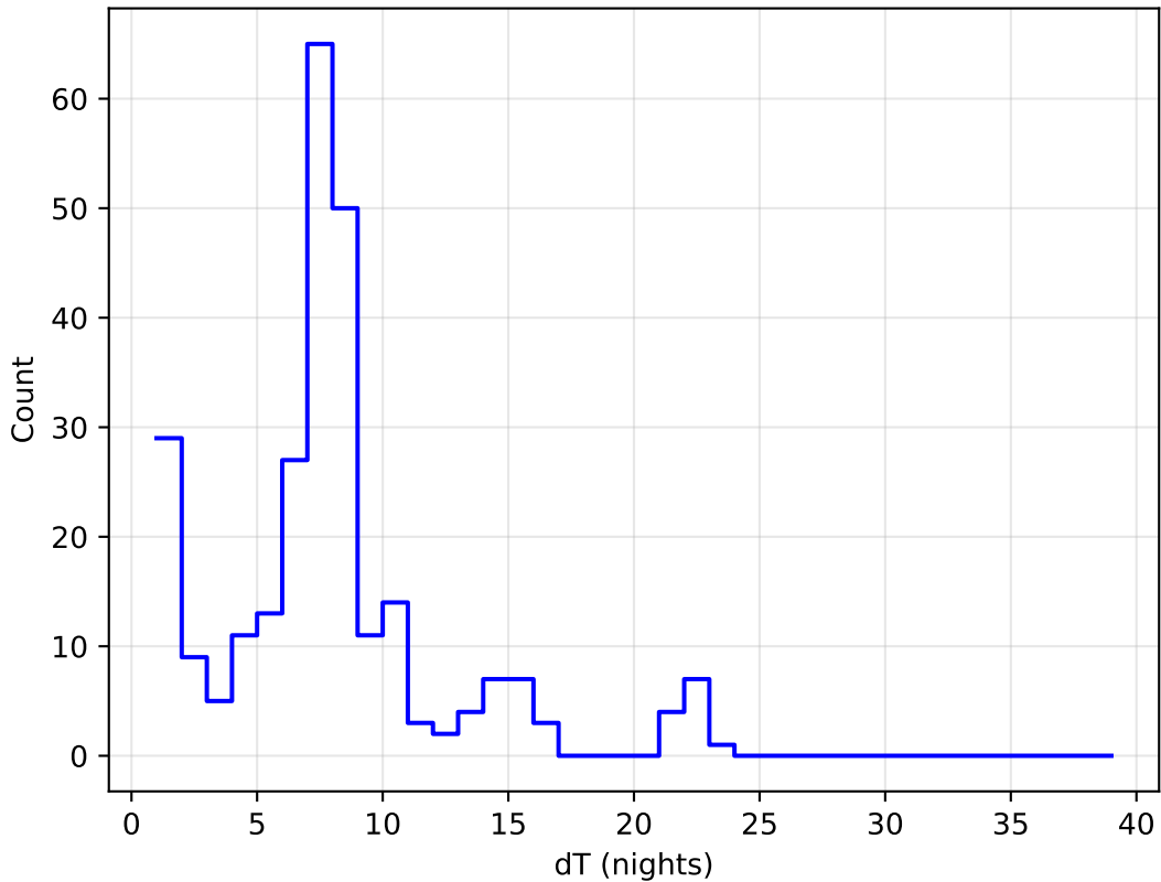
weather_cloudso4v3.4_10yrs all bands: DD:EDFS Delta Nights Histogram
