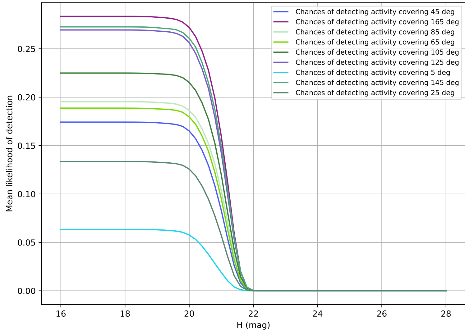
weather_cloudso36v3.4_10yrs Vatira
