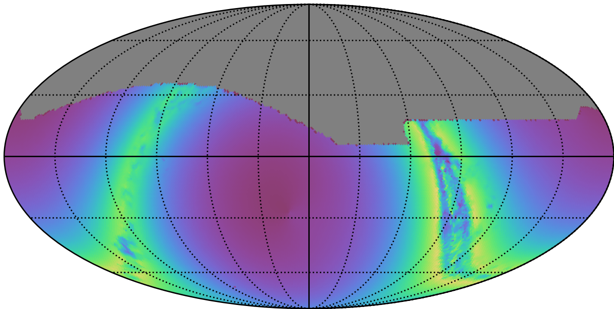
weather_cloudso36v3.4_10yrs : young_stars
