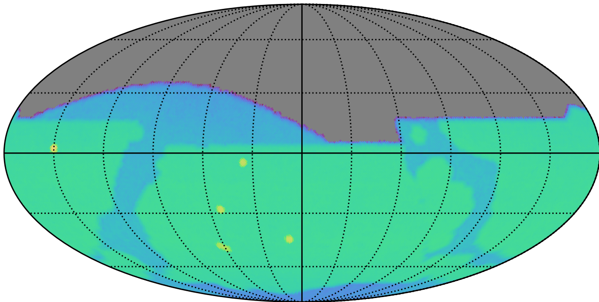
weather_cloudso36v3.4_10yrs i: SurfaceBrightLimit
