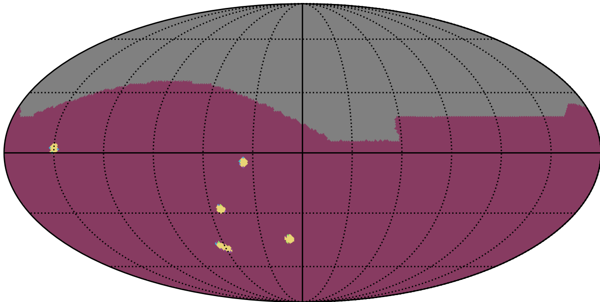
weather_cloudso36v3.4_10yrs : NumberOfQuickRevisits
