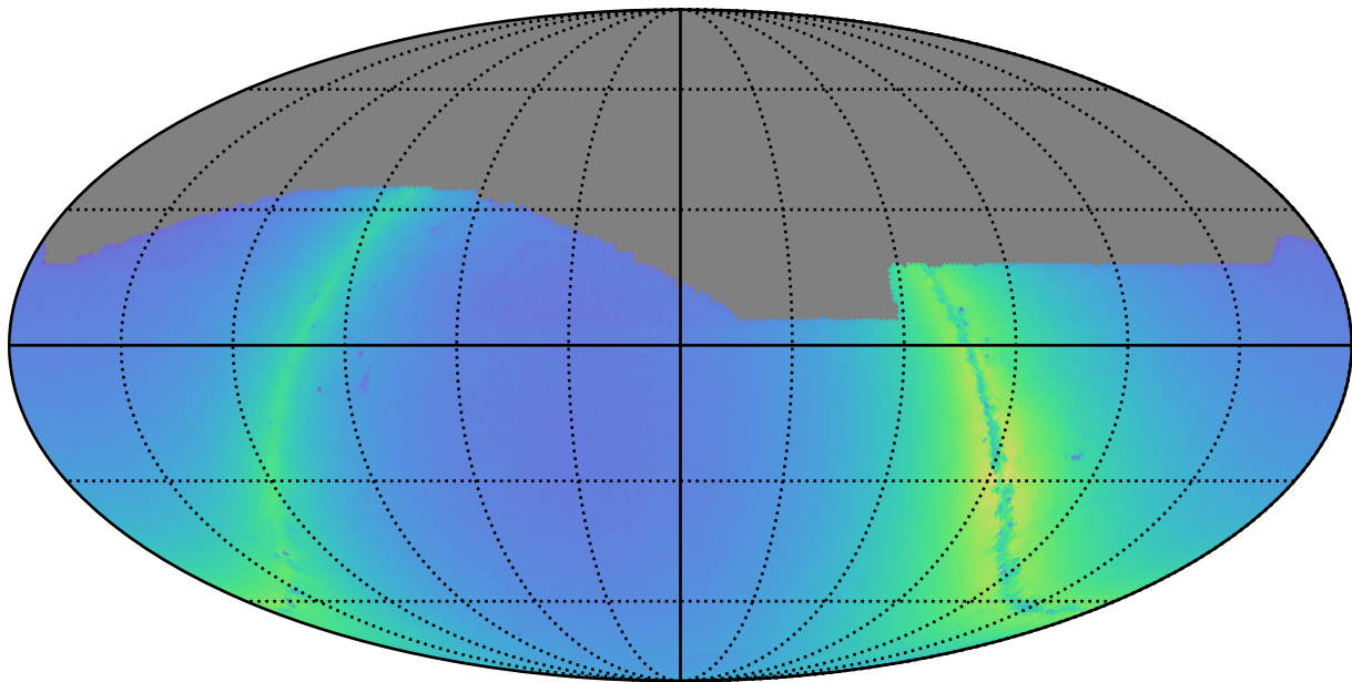
weather_cloudso36v3.4_10yrs z: Nstars_no_crowding
