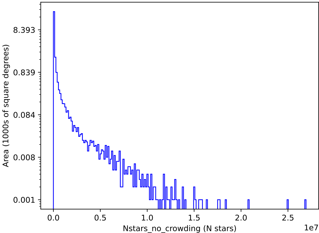
weather_cloudso36v3.4_10yrs z: Nstars_no_crowding
