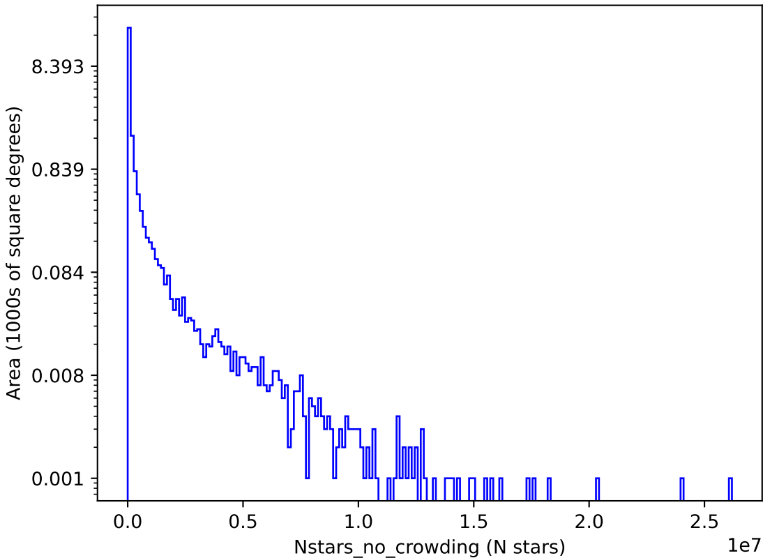
weather_cloudso36v3.4_10yrs y: Nstars_no_crowding
