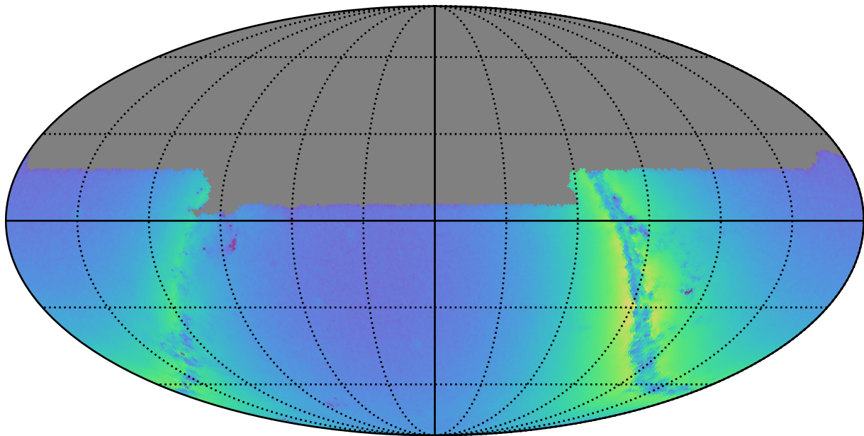
weather_cloudso36v3.4_10yrs u: Nstars_no_crowding
