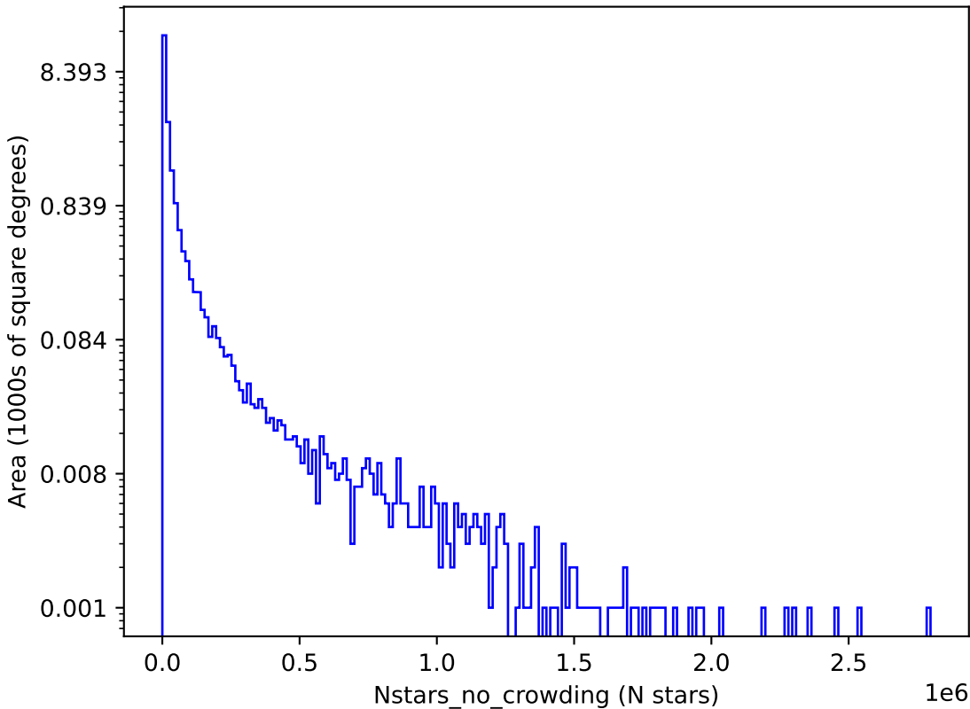
weather_cloudso36v3.4_10yrs u: Nstars_no_crowding
