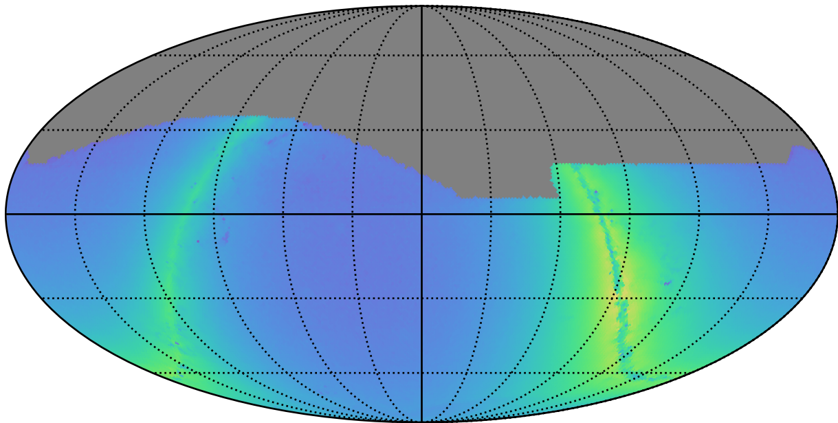
weather_cloudso36v3.4_10yrs r: Nstars_no_crowding
