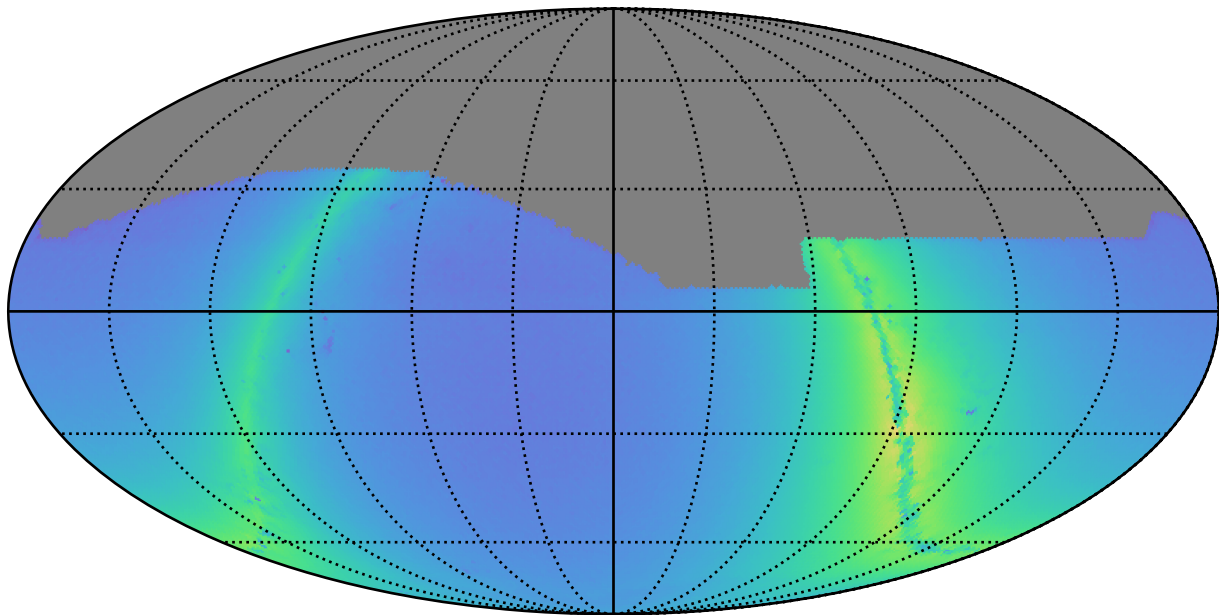
weather_cloudso36v3.4_10yrs i: Nstars_no_crowding
