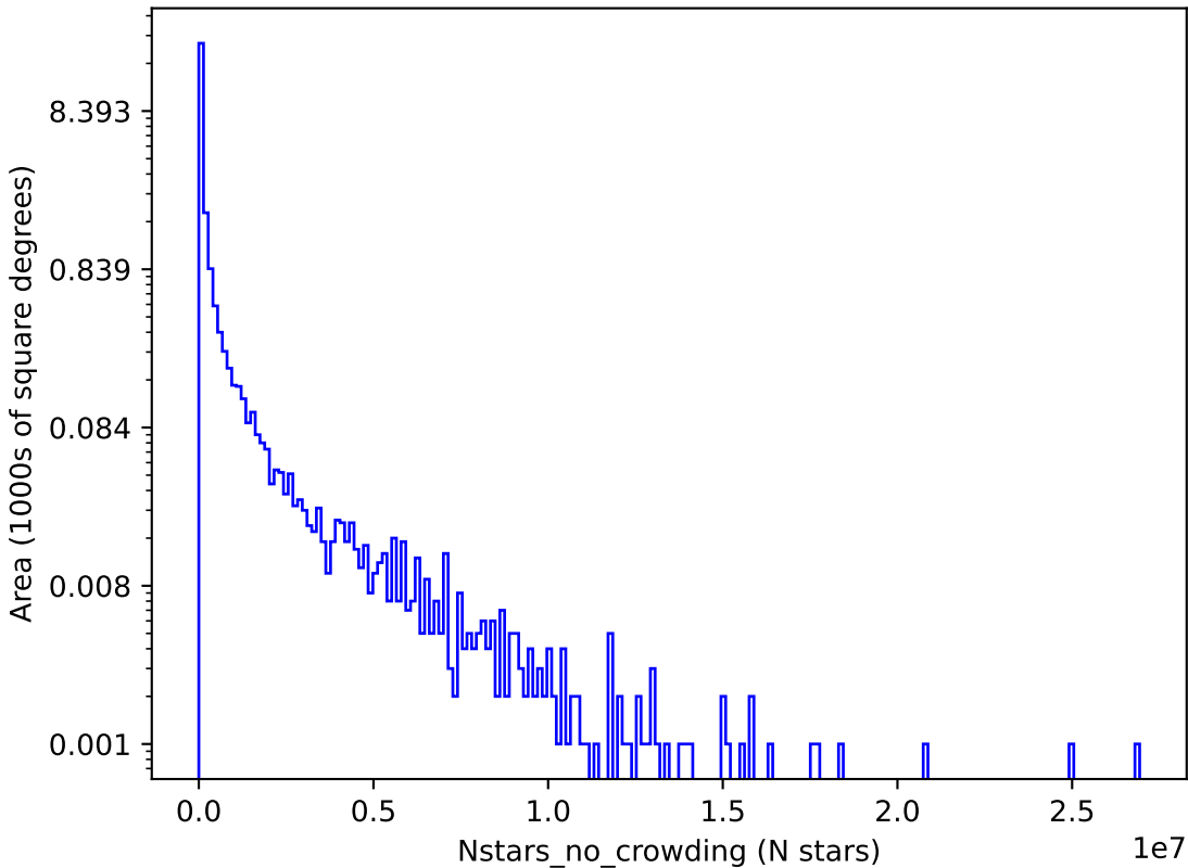
weather_cloudso36v3.4_10yrs i: Nstars_no_crowding
