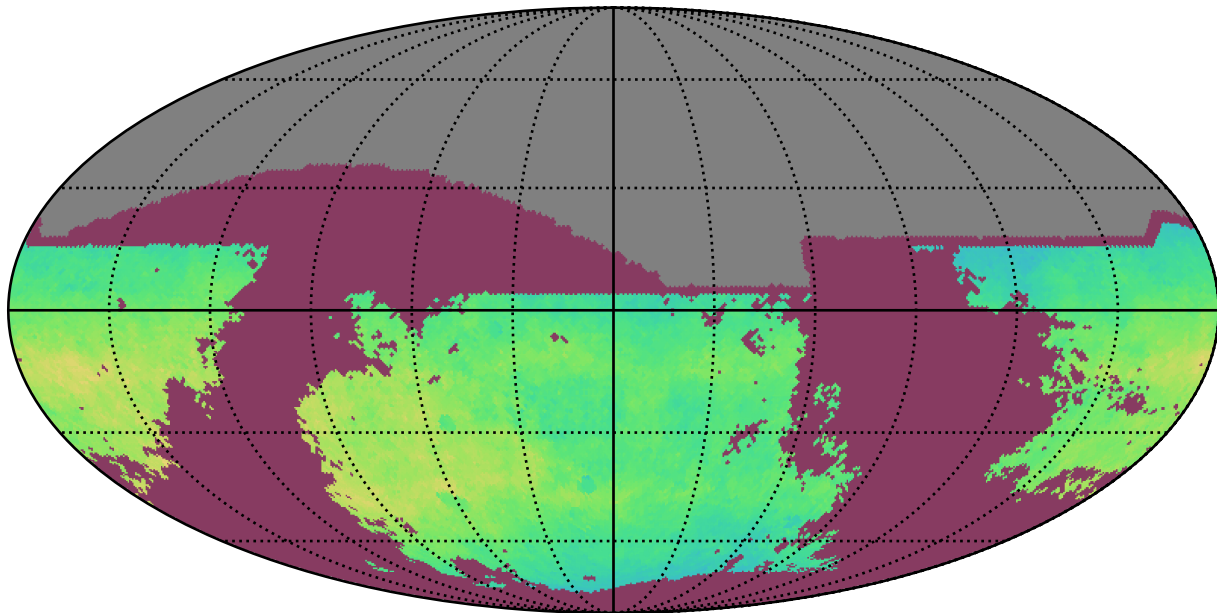
weather_cloudso36v3.4_10yrs i: NgalScale
