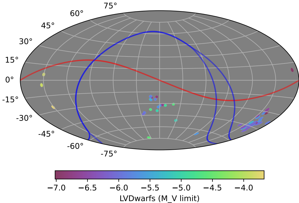
weather_cloudso36v3.4_10yrs gi: LVDwarfs
