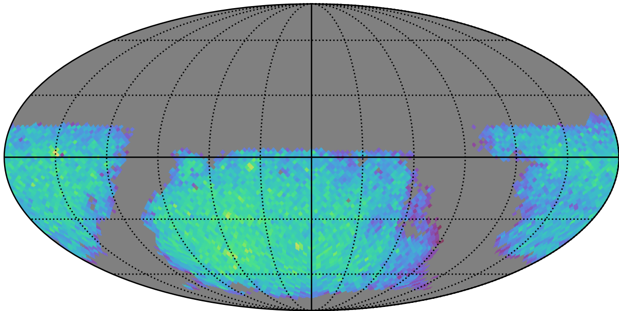
weather_cloudso36v3.4_10yrs gi: LVDwarfs
