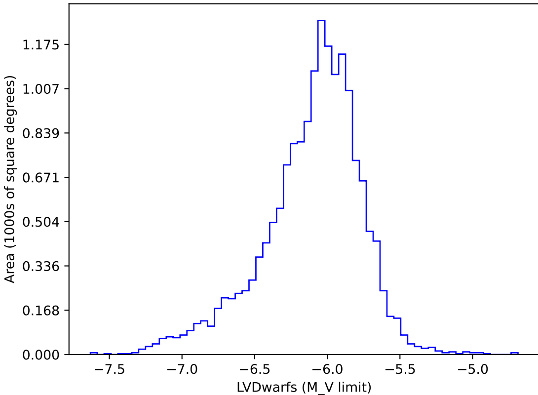
weather_cloudso36v3.4_10yrs gi: LVDwarfs
