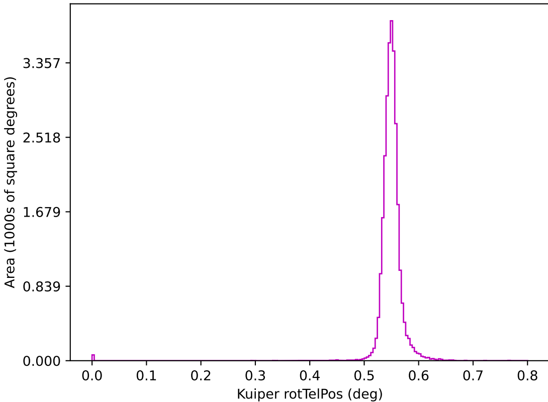
weather_cloudso36v3.4_10yrs z: Kuiper rotTelPos
