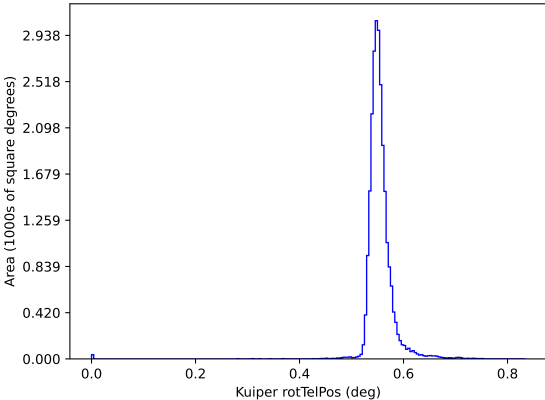
weather_cloudso36v3.4_10yrs y: Kuiper rotTelPos
