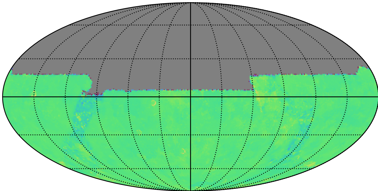
weather_cloudso36v3.4_10yrs u: Kuiper rotTelPos
