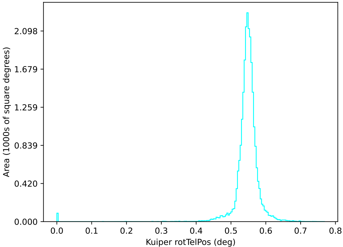
weather_cloudso36v3.4_10yrs u: Kuiper rotTelPos
