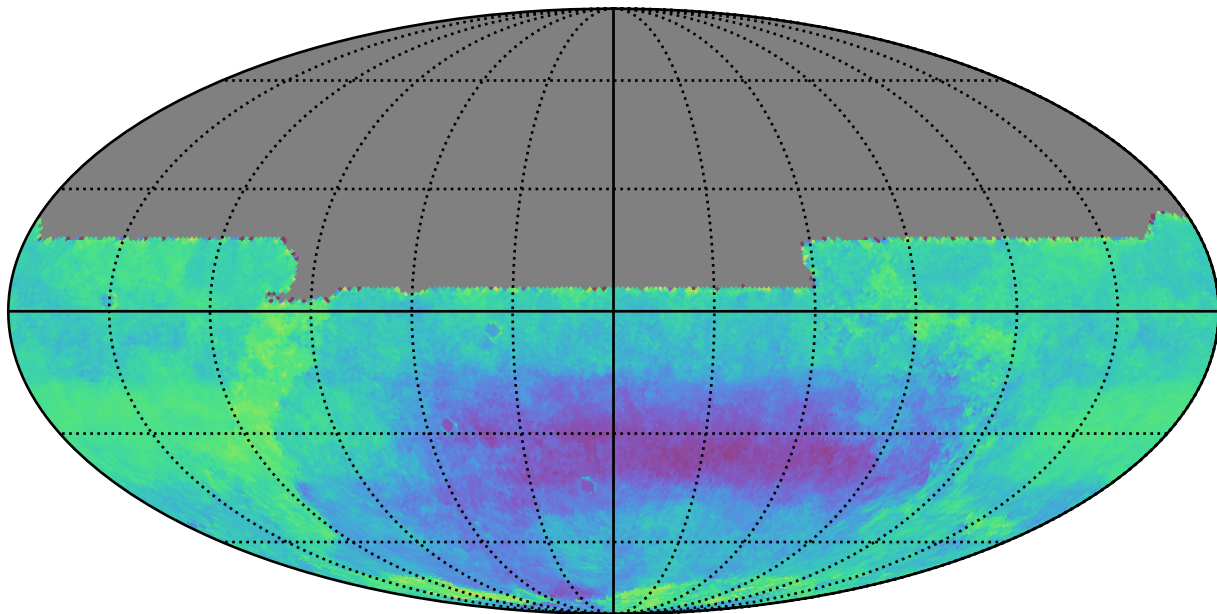
weather_cloudso36v3.4_10yrs y: Kuiper rotSkyPos
