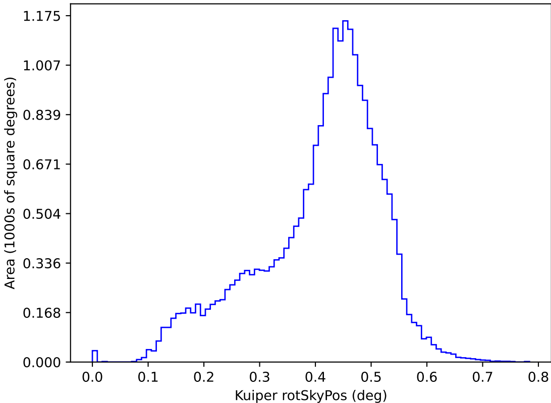
weather_cloudso36v3.4_10yrs y: Kuiper rotSkyPos
