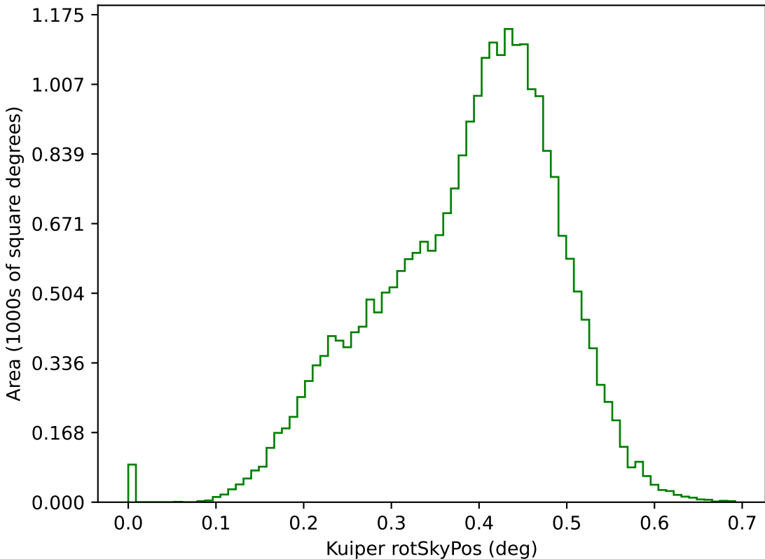
weather_cloudso36v3.4_10yrs g: Kuiper rotSkyPos
