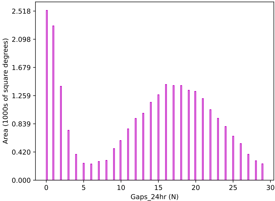
weather_cloudso36v3.4_10yrs z band: Gaps_24hr
