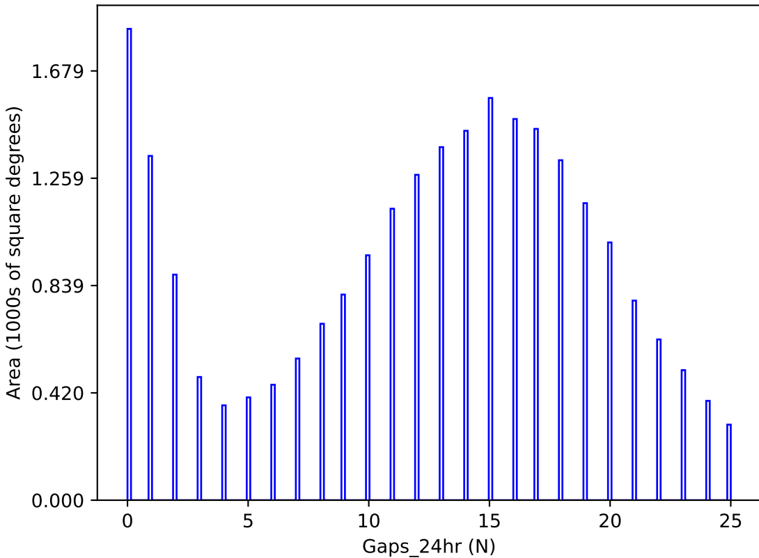
weather_cloudso36v3.4_10yrs y band: Gaps_24hr
