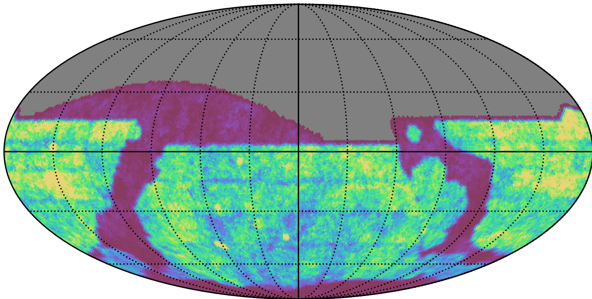
weather_cloudso36v3.4_10yrs r band: Gaps_24hr
