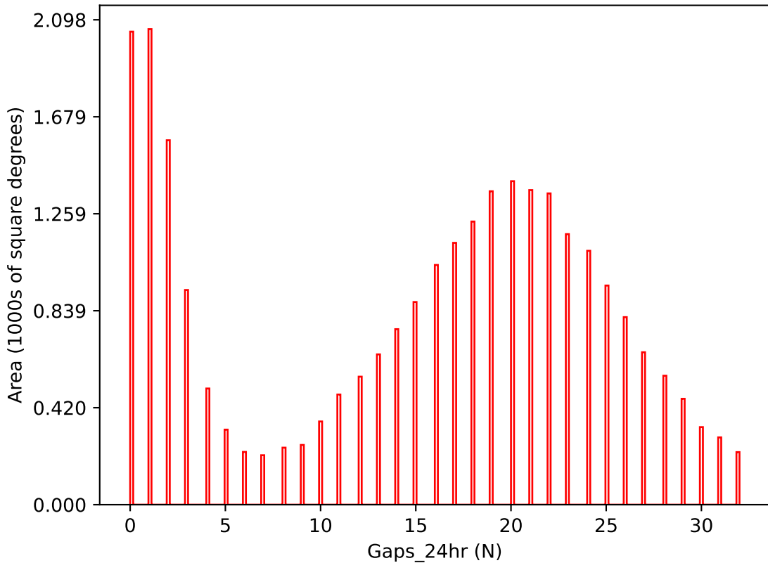
weather_cloudso36v3.4_10yrs i band: Gaps_24hr
