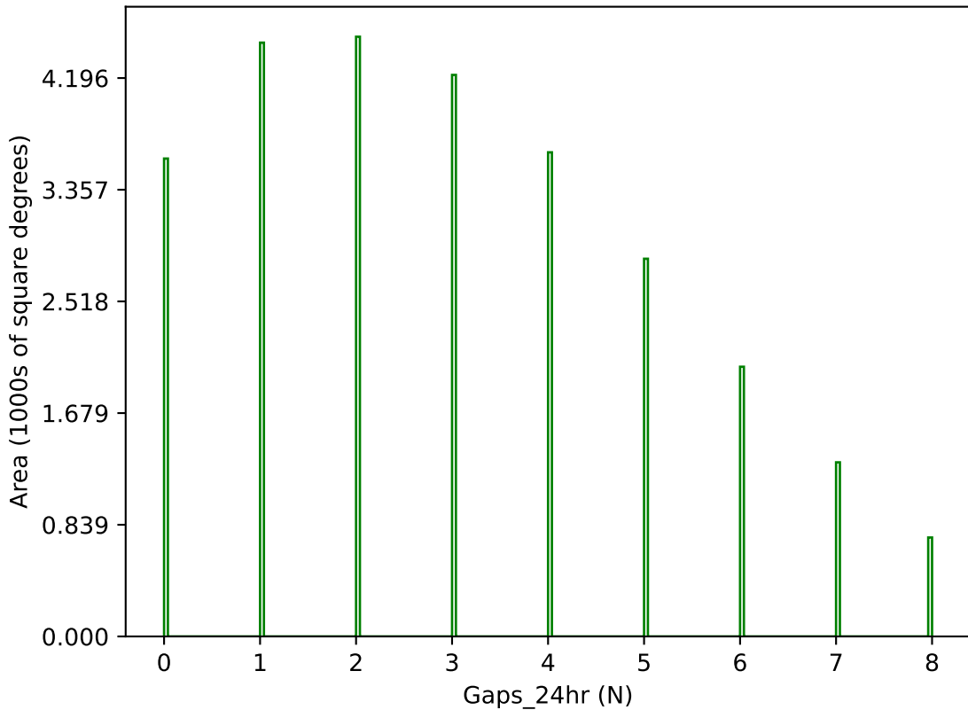
weather_cloudso36v3.4_10yrs g band: Gaps_24hr
