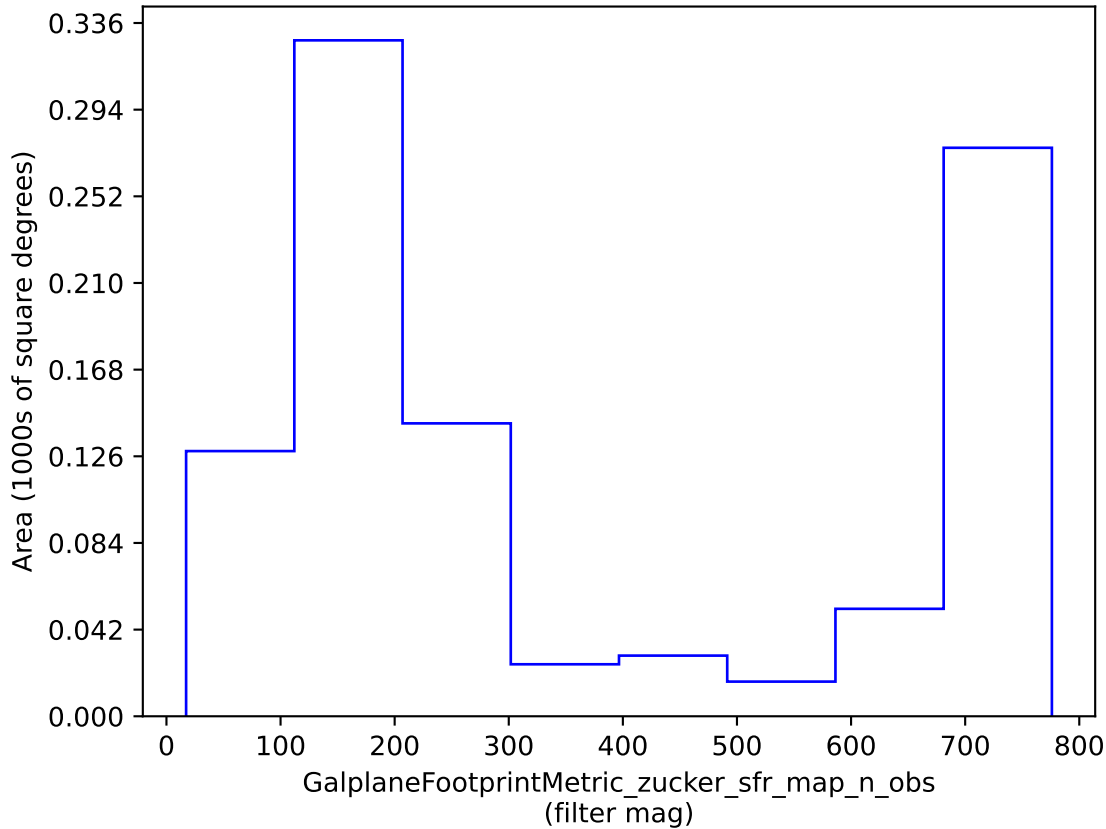
weather_cloudso36v3.4_10yrs : GalplaneFootprintMetric_zucker_sfr_map_n_obs
