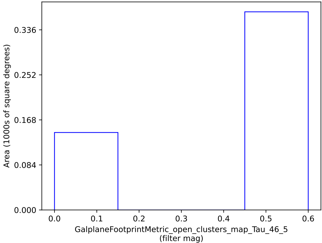
weather_cloudso36v3.4_10yrs : GalplaneFootprintMetric_open_clusters_map_Tau_46_5
