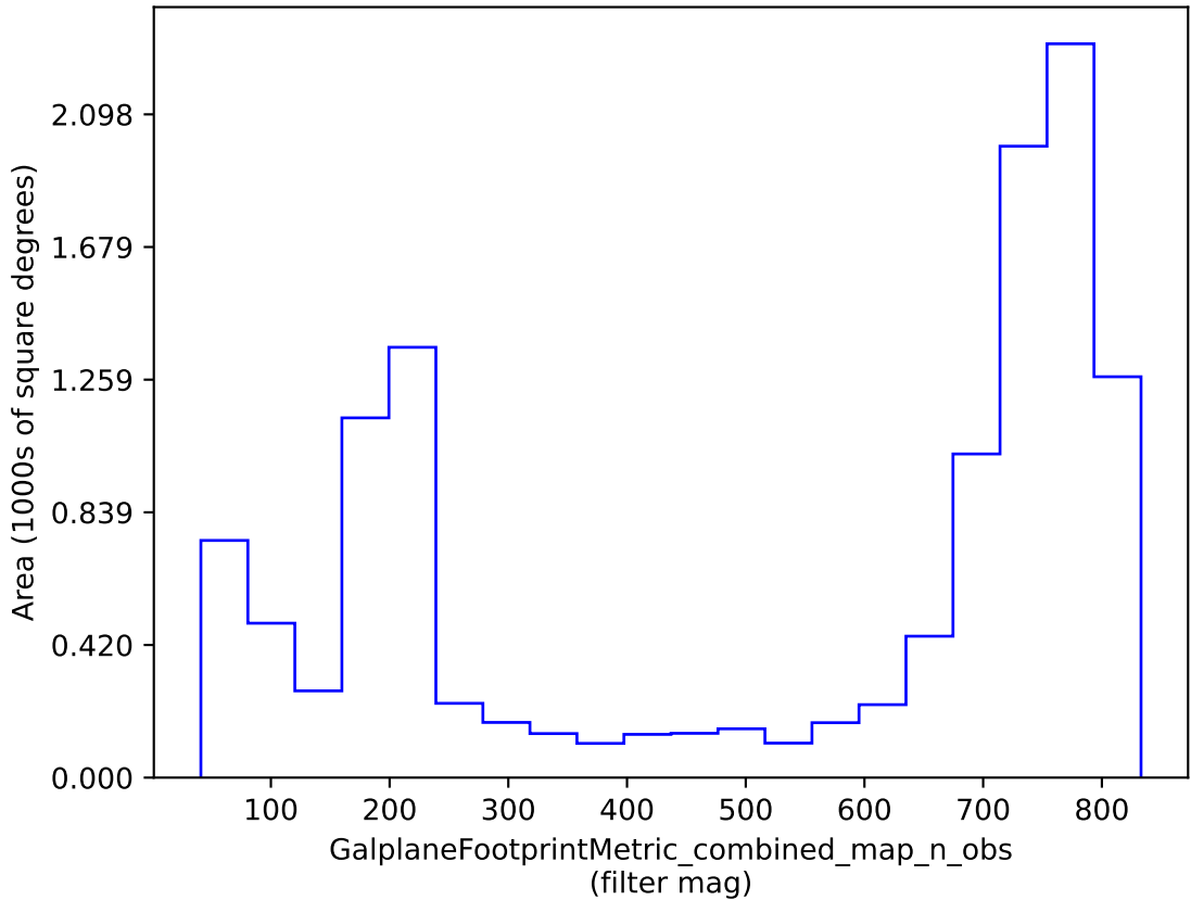
weather_cloudso36v3.4_10yrs : GalplaneFootprintMetric_combined_map_n_obs
