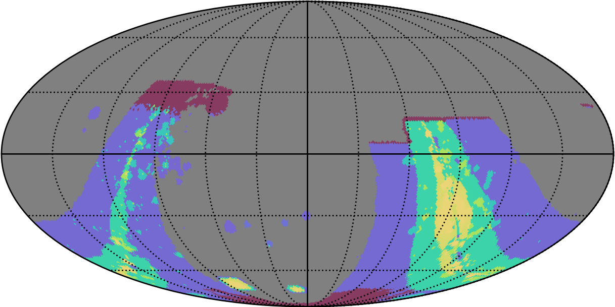
weather_cloudso36v3.4_10yrs : GalplaneFootprintMetric_combined_map_Tau_46_5
