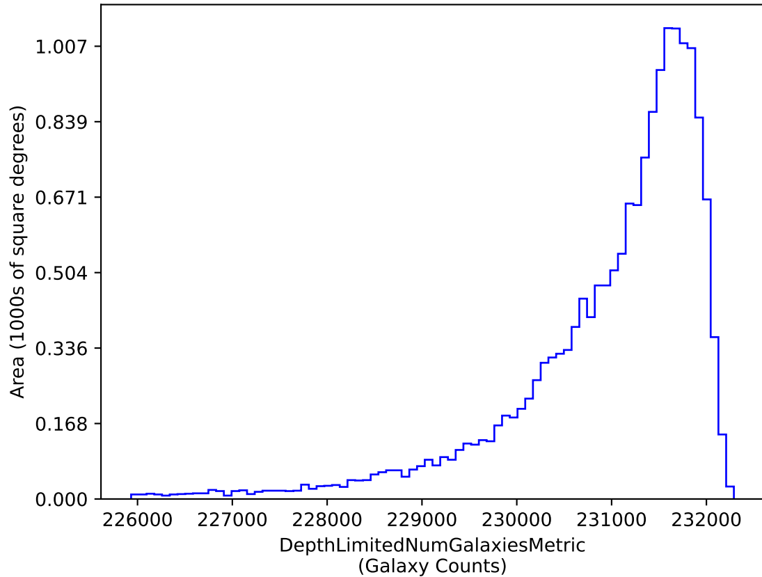
weather_cloudso36v3.4_10yrs i band galaxies non-DD: DepthLimitedNumGalaxiesMetric
