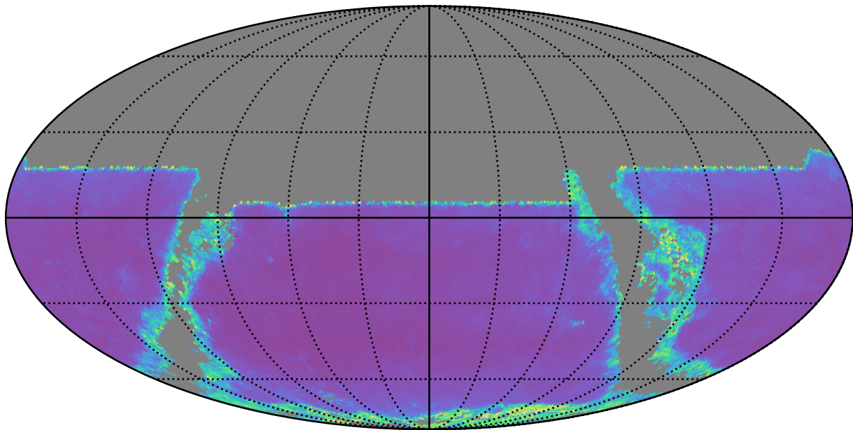
weather_cloudso36v3.4_10yrs y band: AGN SF_uncert
