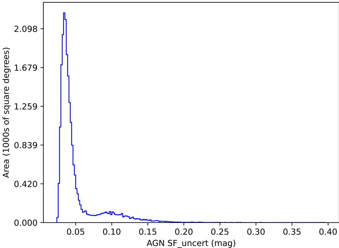
weather_cloudso36v3.4_10yrs y band: AGN SF_uncert
