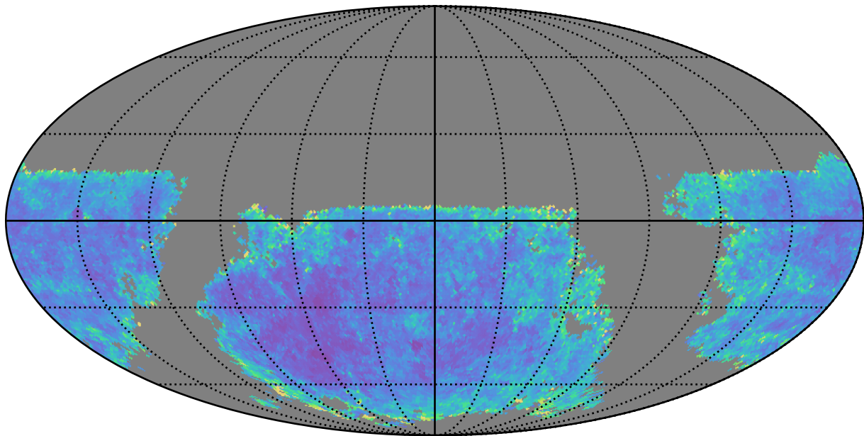
weather_cloudso36v3.4_10yrs u band: AGN SF_uncert
