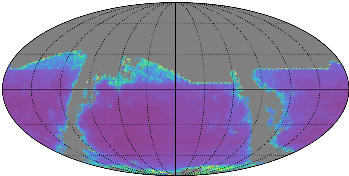
weather_cloudso36v3.4_10yrs r band: AGN SF_uncert
